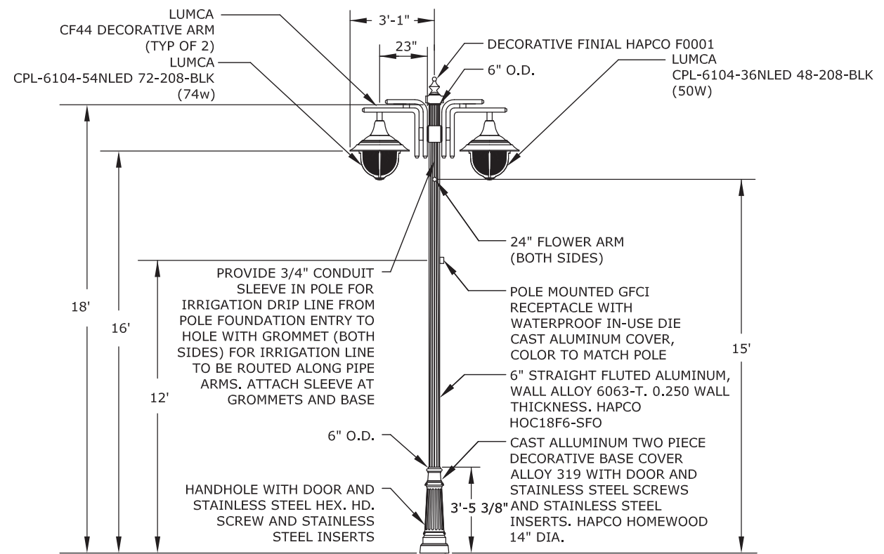
TYPE P2C
