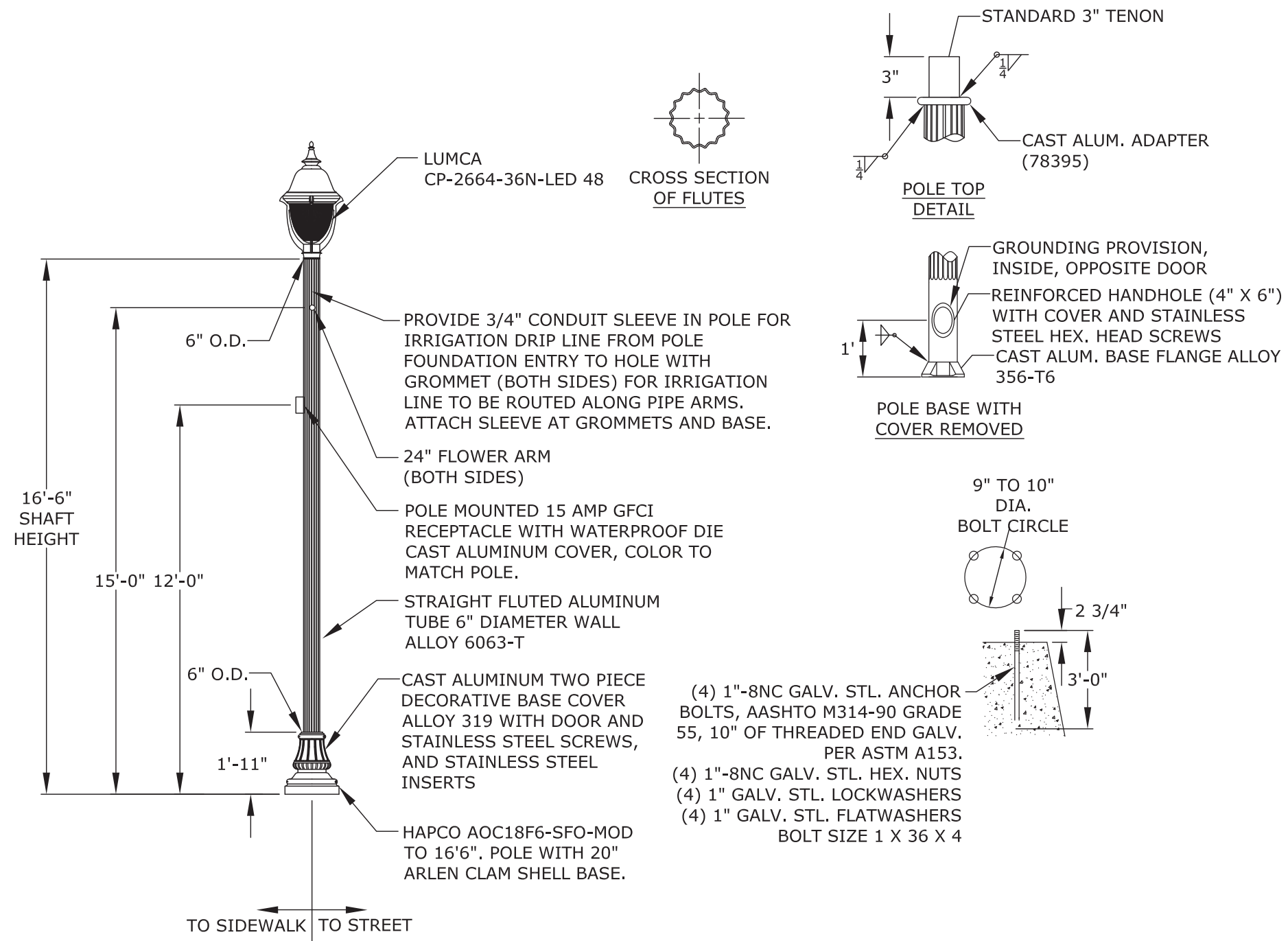
TYPE P1A
