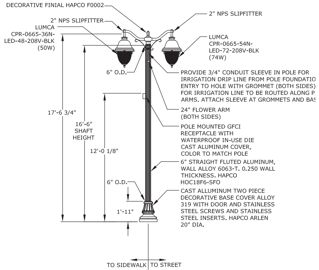
TYPE P2B
